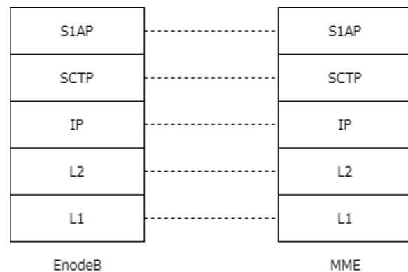
Fig. 1. S1: E-UTRAN-MME Interface
