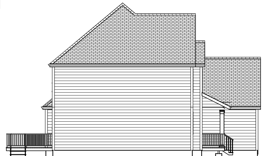
Elevation 4
