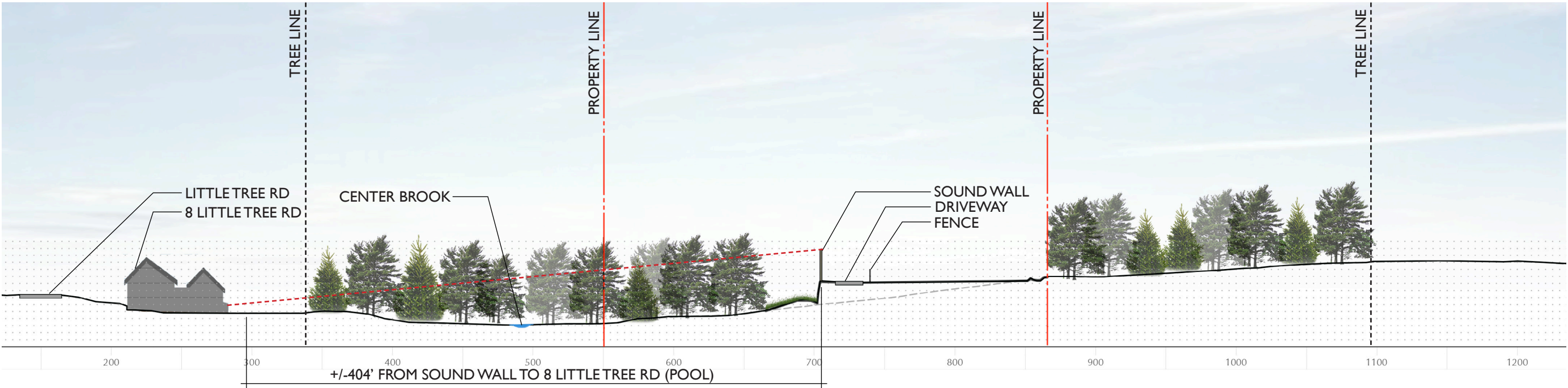
SECTION A-A
