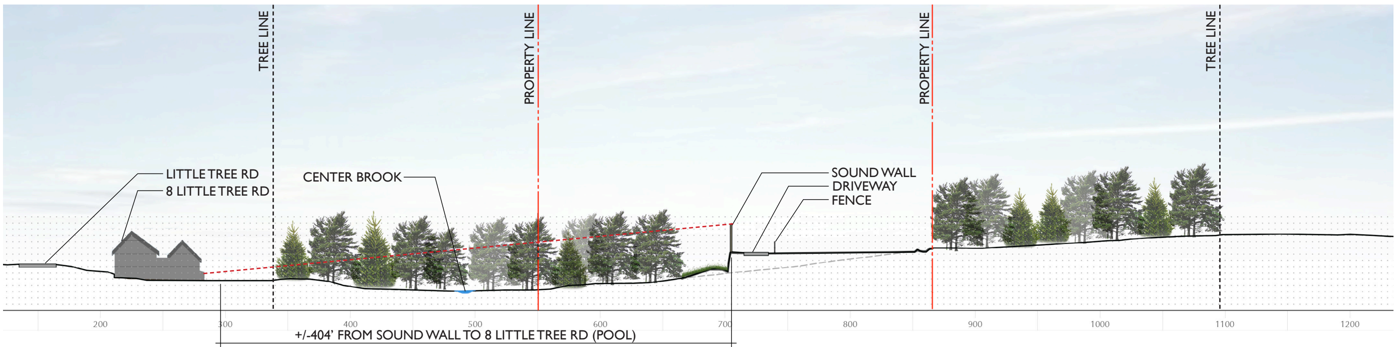
SECTION A-A
