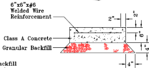
Sec. A-A
