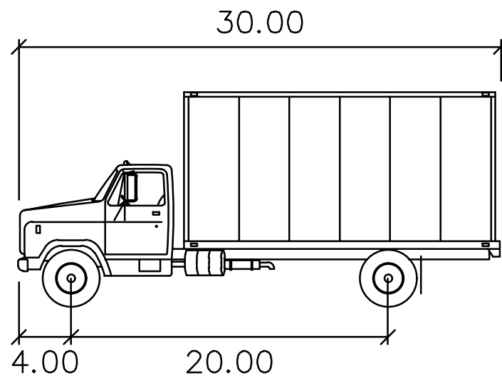
SU-30
