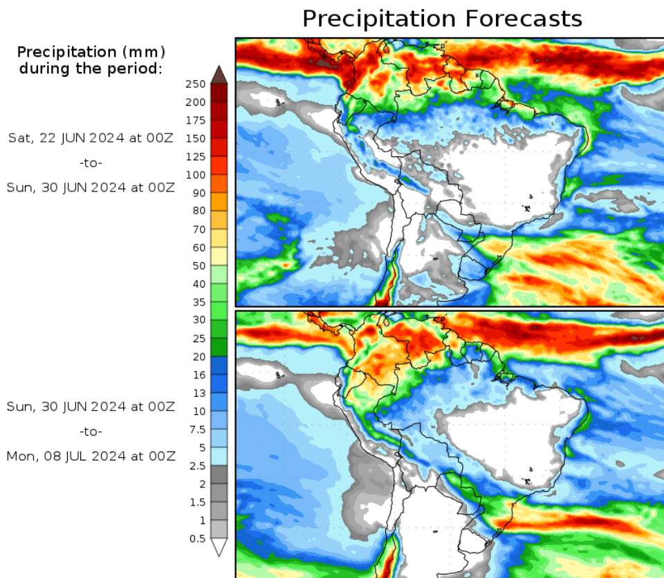
Available at: http://wxmaps.org/pix/prec8
