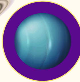
Uranus
