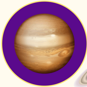
Jupiter
