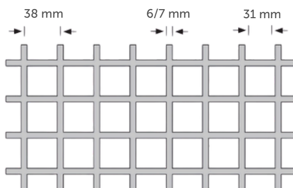
Draufsicht
