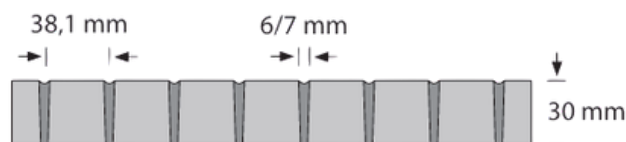
Seitenansicht
