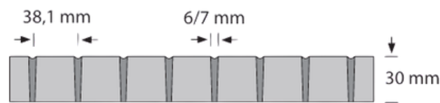
Seitenansicht
