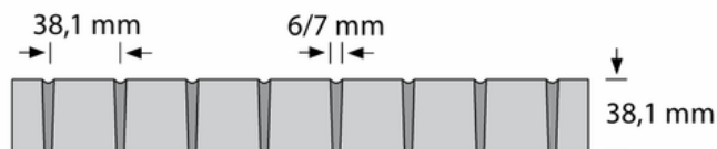
Seitenansicht
