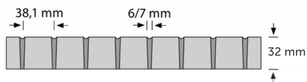
Seitenansicht
