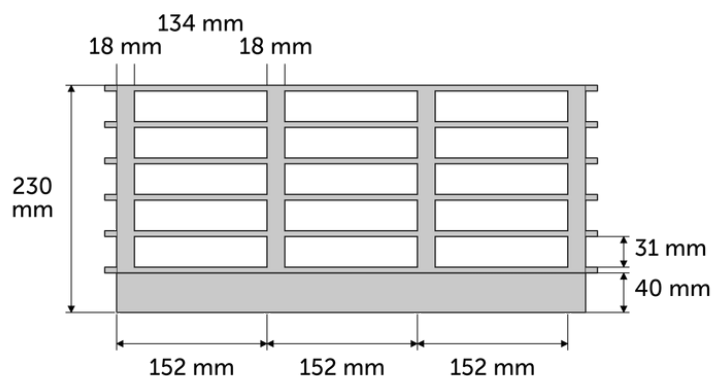
Draufsicht
