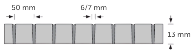
Zij-aanzicht
