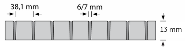
Zij-aanzicht
