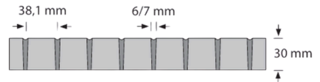
Zij-aanzicht
