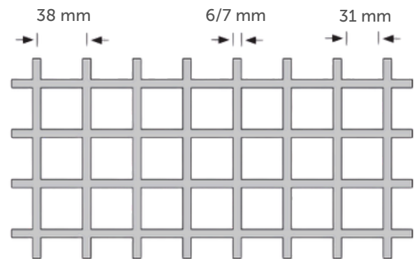
Bovenaanzicht
