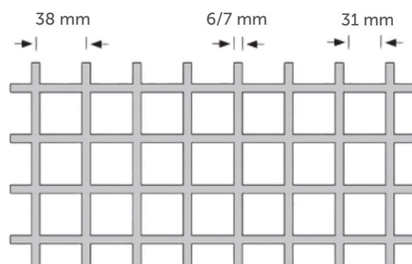
Bovenaanzicht
