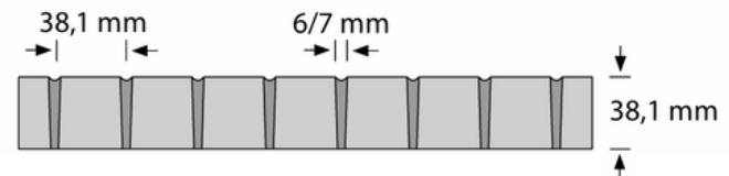
Zij-aanzicht
