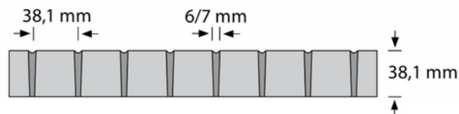
Zij-aanzicht
