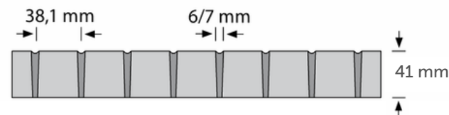
Zij-aanzicht
