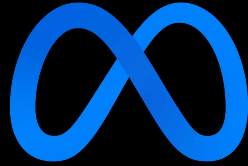
Llama-3 Model
