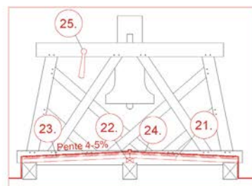
COUPE EST-OUEST
