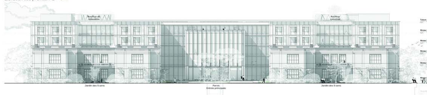
Elevation sud | Pavillon E - 1/100
