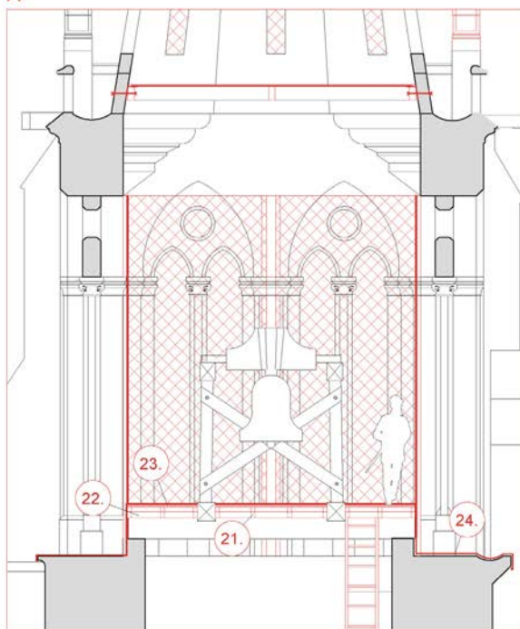
COUPE NORD-SUD
