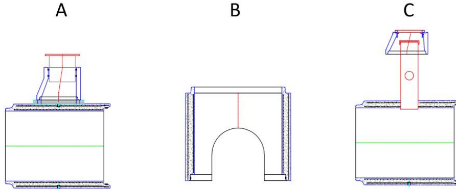
Kuva 1. Satula kaivotyypit. A = putken päälle tehtaalla asennettu, B = renkaaseen avarrettu ura, C = putken porattava nousuputki tarkastusluukulla ja suojakartiolla jossa valurautakansisto.
