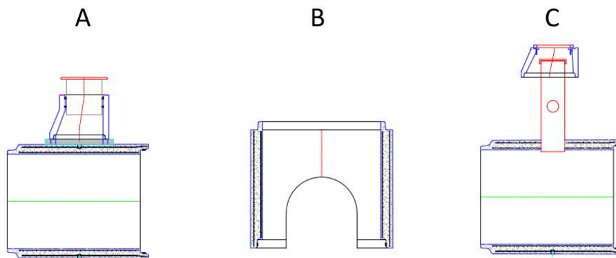
Kuva 1. Satula kaivotyypit. A = putken päälle tehtaalla asennettu, B = renkaaseen avarrettu ura, C = putkeen porattava nousuputki tarkastusluukulla ja suojakartiolla jossa valurautakanansisto.
