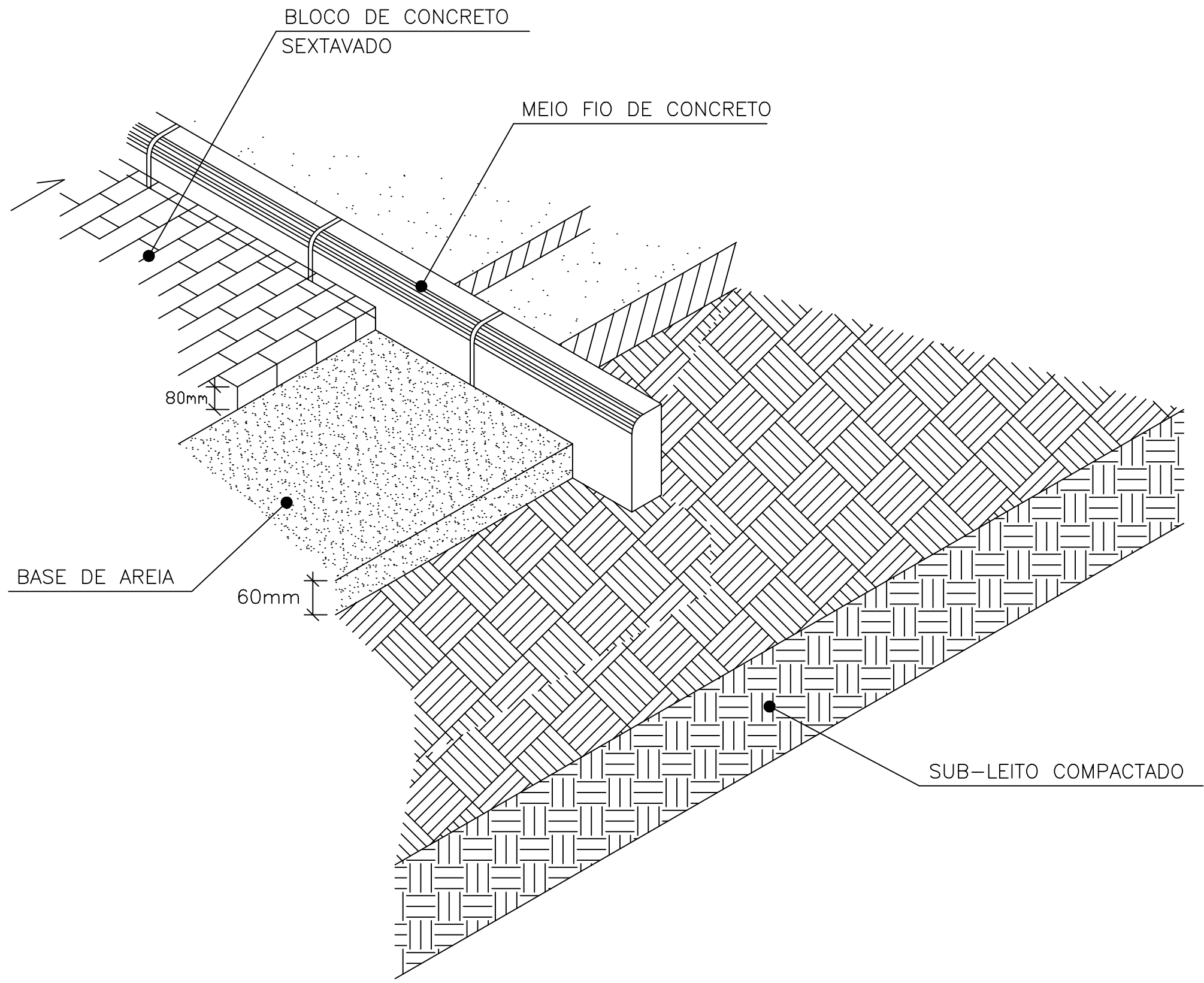
DETALHE EM PERSPECTIVA DE CALÇAMENTO ESC. : SEM ESCALA
