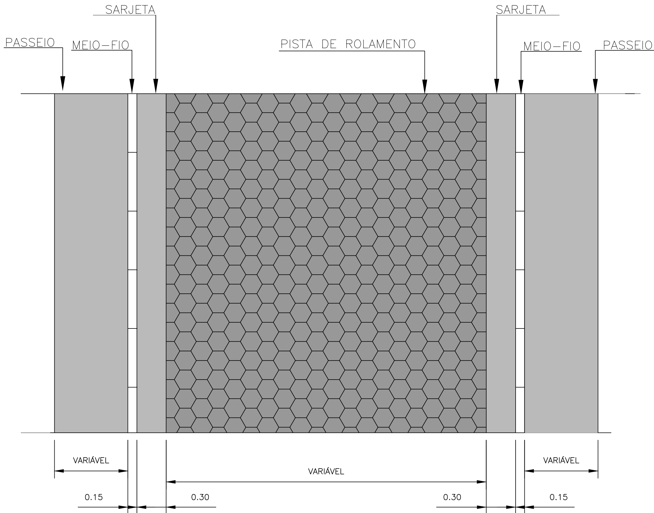
PLANTA TIPO DA PAVIMENTAÇÃO ESC. 1:50
