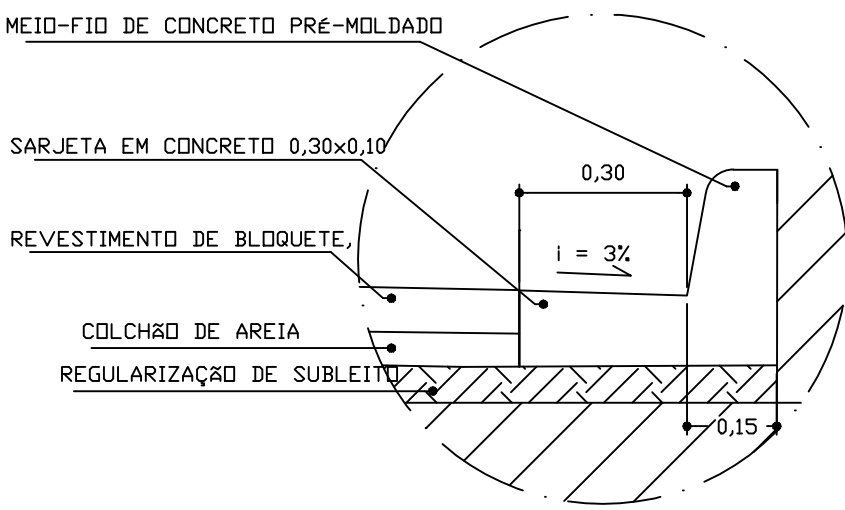
DETALHE 01 - MEIO-FIO E SARJETA - BLOQUETE
