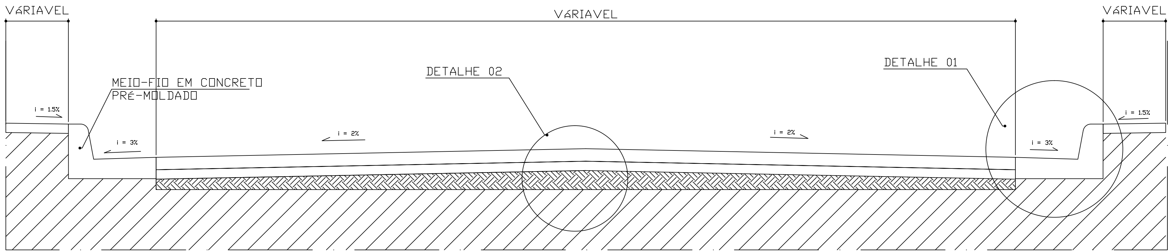
SEÇÃO TIPO ESCALA 1/20
