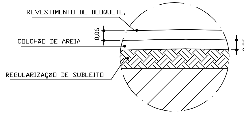
DETALHE 02 - CORTE CAMADAS BLOQUETE
