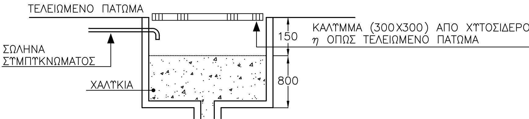
ΛΕΠΤΟΜΕΡΕΙΑ 1 ΑΠΟΡΡΟΦΗΤΙΚΟΤ ΛΑΚΚΟΤ ΣΤΥΠΤΚΝΩΜΑΤΩΝ
