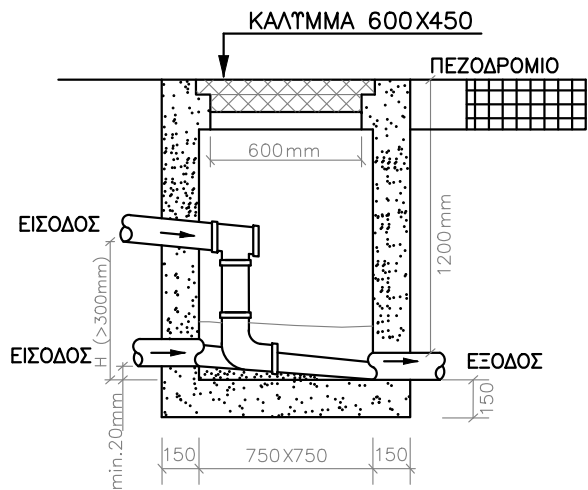
ΦΡΕΑΤΙΟ ΣΤΗΝΔΕΣΗΣ (750mm X 750mm)
