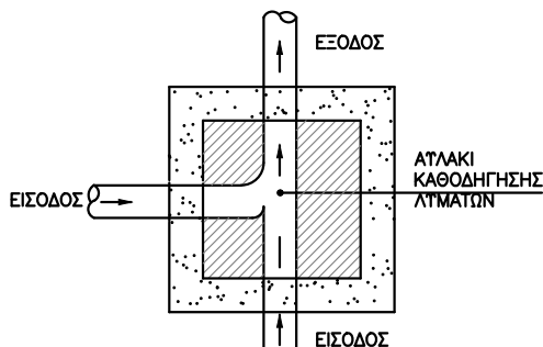
ΤΥΠΙΚΗ ΚΑΤΟΨΗ ΦΡΕΑΤΙΩΝ (ΜΕ ΔΥΟ ΕΙΣΟΔΟΥΣ)
