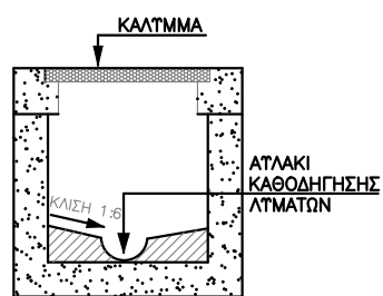
ΤΥΠΙΚΗ ΤΟΜΗ ΦΡΕΑΤΙΩΝ
