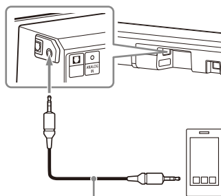
Câble audio analogique (non fourni) Smartphone, WALKMAN®, autres dispositifs audio, etc.
