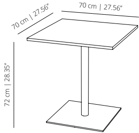
ST72C70_ table 70x70 | table 27 61/64 x 27 61/64
