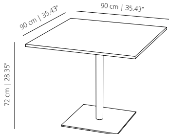
ST72C90_ table 90x90 | table 35 7/16 x 35 7/16
