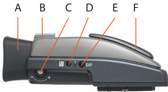
A. Œilleton en caoutchouc B. Sabot C. Molette de réglage de dioptrie
