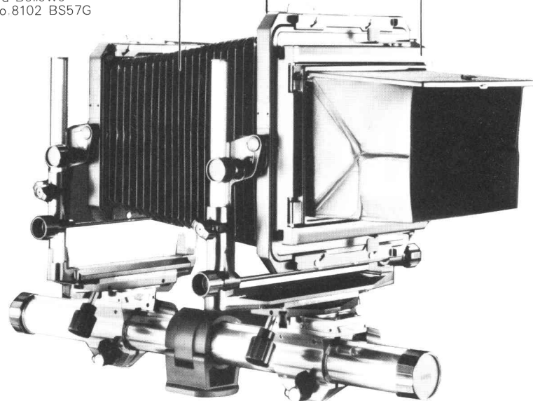
標準ジャバラ 57G Standard Bellows Cat. No.8102 BS57G
