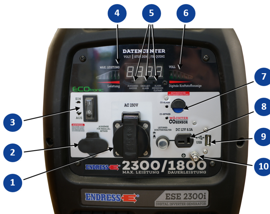
Fig. 6-4 Komponenter på manöverpanelen
