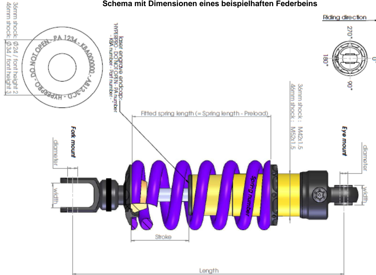
Schema mit Dimensionen eines beispielhaften Federbeins
