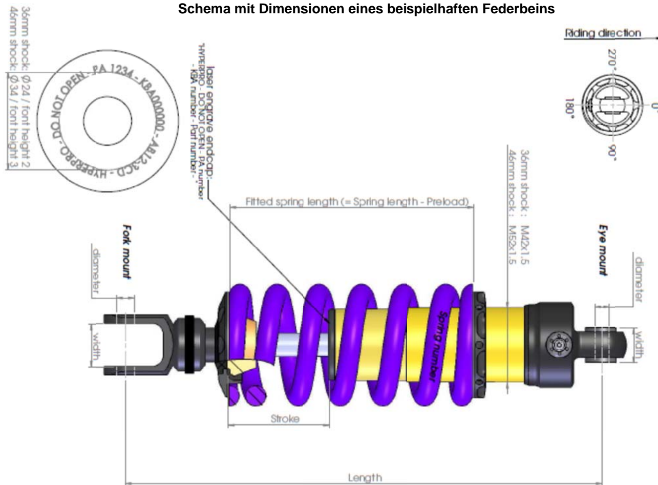
Schema mit Dimensionen eines beispielhaften Federbeins
