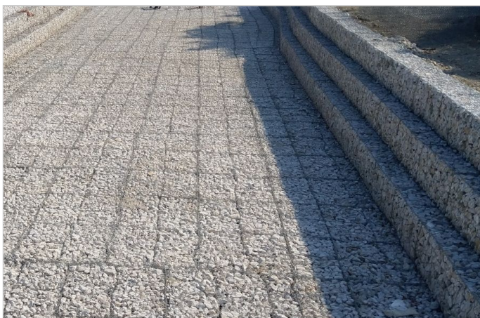
Ολοκλήρωση εργασιών τοποθέτησης, πλήρωσης & συρραφής συρματοκιβωτίων
