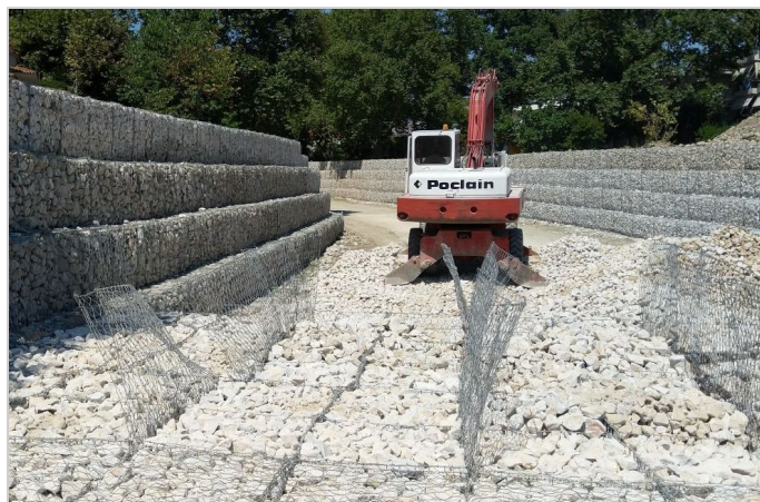
Διαδικασία πλήρωσης συρματοκιβωτίων
