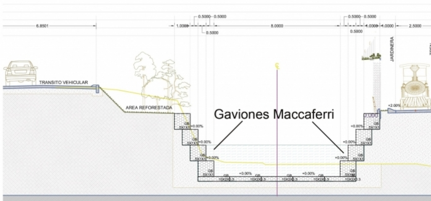
Representación esquemática
