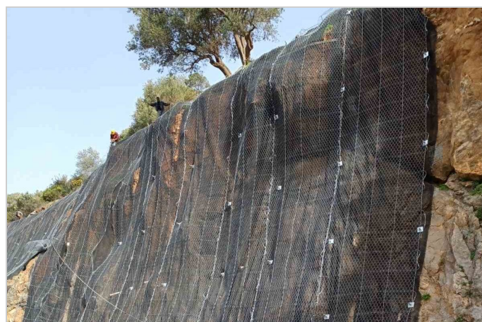
ΠΛΗΡΩΣ ΑΓΚΥΡΟΥΜΕΝΟ ΠΛΕΓΜΑ MACARMOUR 60x60 ΣΤΗ ΦΑΣΗ ΤΗΣ ΤΟΠΟΘΕΤΗΣΗΣ
