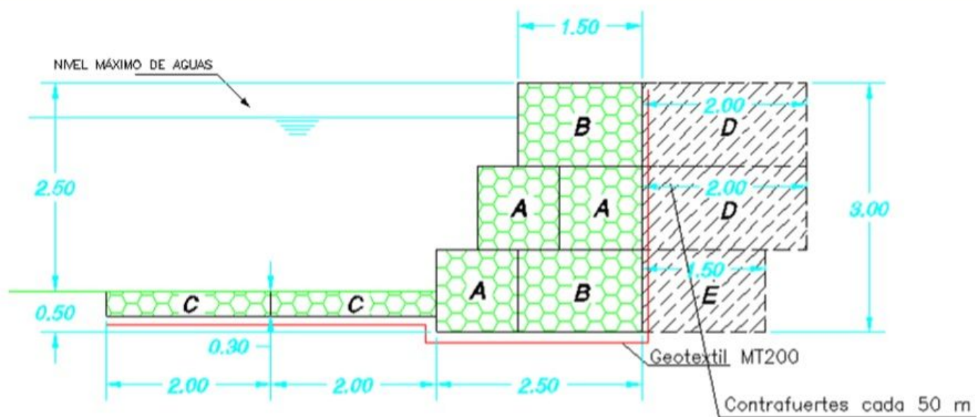
(Sección transversal típica)
