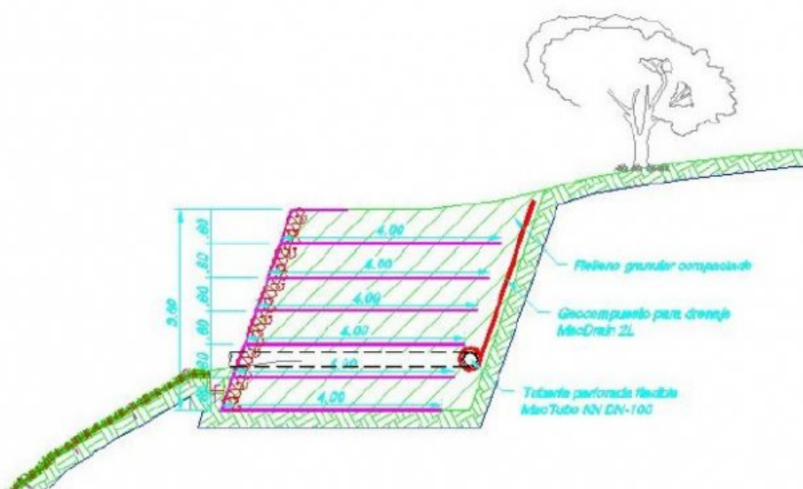
Sección Típica Terramesh Verde
