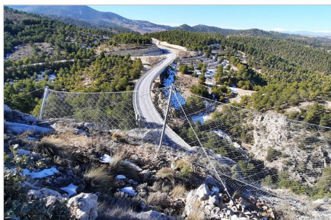
Barrera dinámica RB 750
