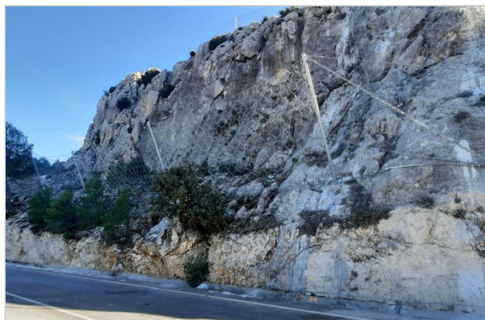
Vista Barreras RB 1000 y RB 750 desde lado monte
