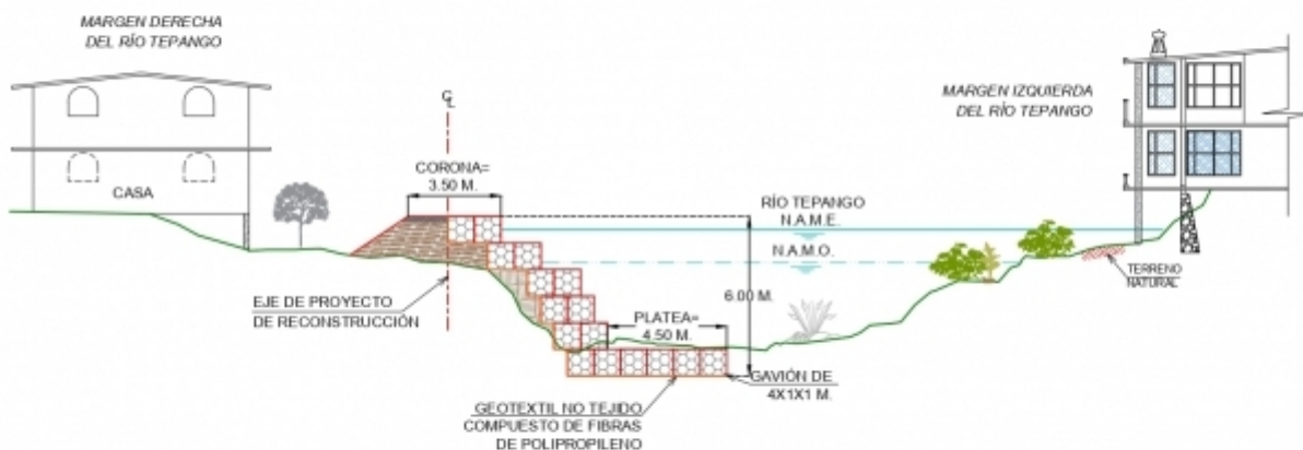
SECCIÓN TIPO DE LA RECONSTRUCCIÓN DE LAS MARGENES DEL RÍO TEPANGO DEL KM. 1+050 AL KM. 1+080 (L=30.00 M.)
