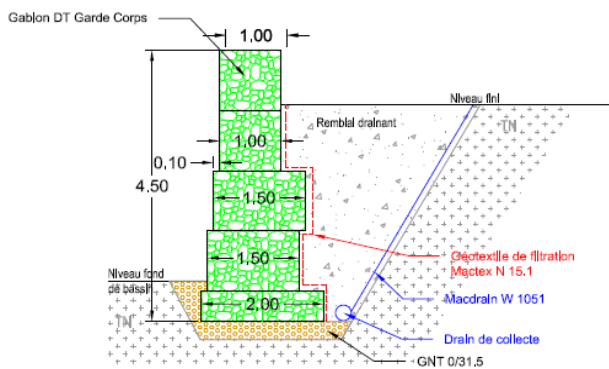
Coupe du mur
