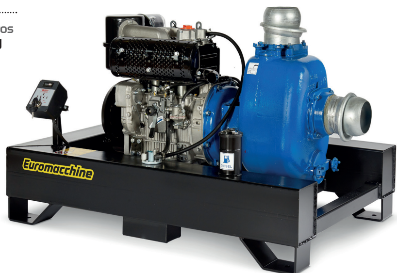
Dízelmotoros SZIVATTYÚ EGYSÉG 150 m 3 /h
