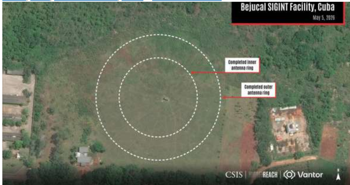
La nueva y extensa red circular de antenas construida en Bejucal, al sur de La Habana. Foto CSIS
