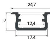
CORTE 18 mm
