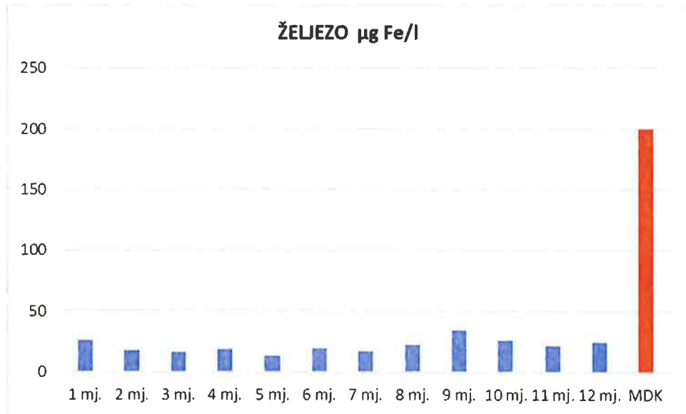
Grafički prikaz koncentracije željeza na ulazu u vodoopskrbnu mrežu tijekom 2024. god.
