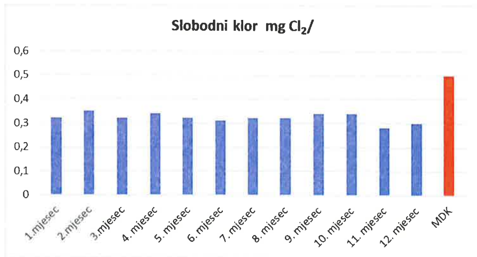
Grafički prikaz koncentracije slobodnog klora na ulazu u gradsku vodoopskrbnu mrežu tijekom 2024. god.
