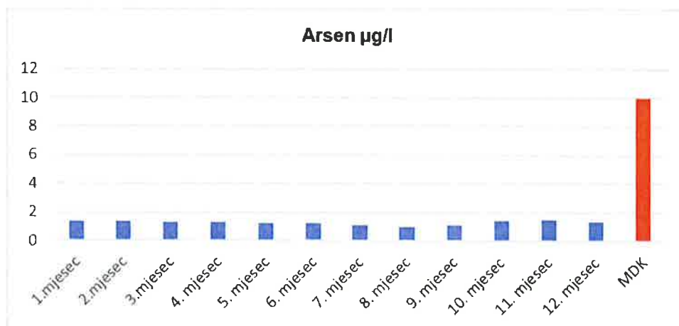
Grafički prikaz koncentracije arsena na ulazu u gradsku vodoopskrbnu mrežu tijekom 2024.god.
