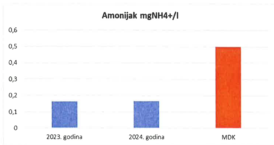
Usporedni grafički prikaz koncentracije amonija u vodi uzorkovanoj na ulazu u gradsku vodoopskrbnu mrežu u Dalju (2023-2024. god.)
