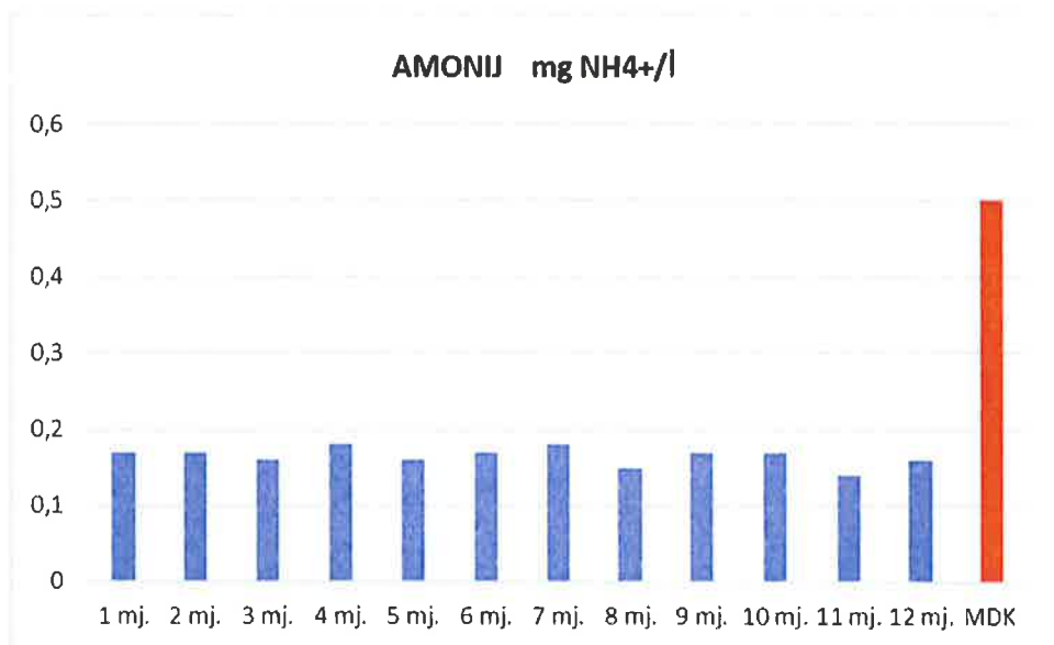
Grafički prikaz koncentracije amonija na ulazu u vodoopskrbnu mrežu tijekom 2024. god.
