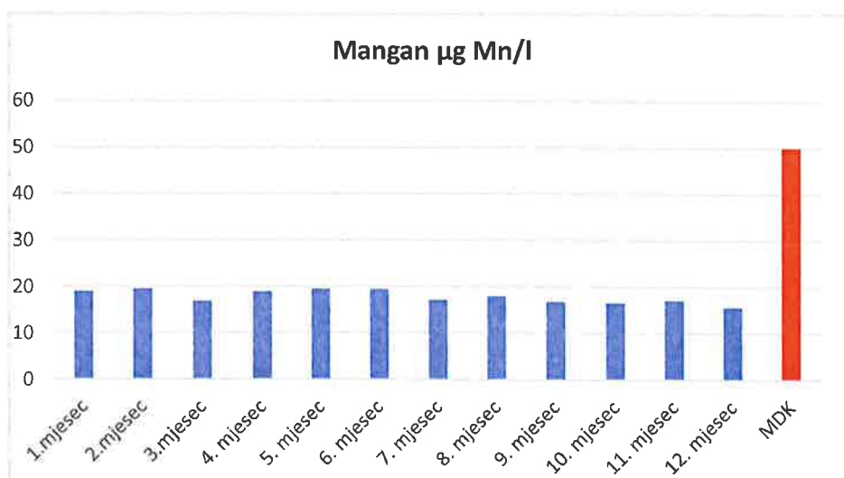
Grafički prikaz koncentracije mangana na ulazu u gradsku vodoopskrbnu mrežu tijekom 2024. god.
