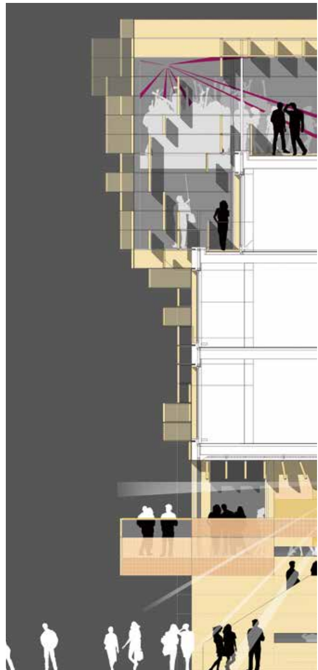
Fassadenschnitt
