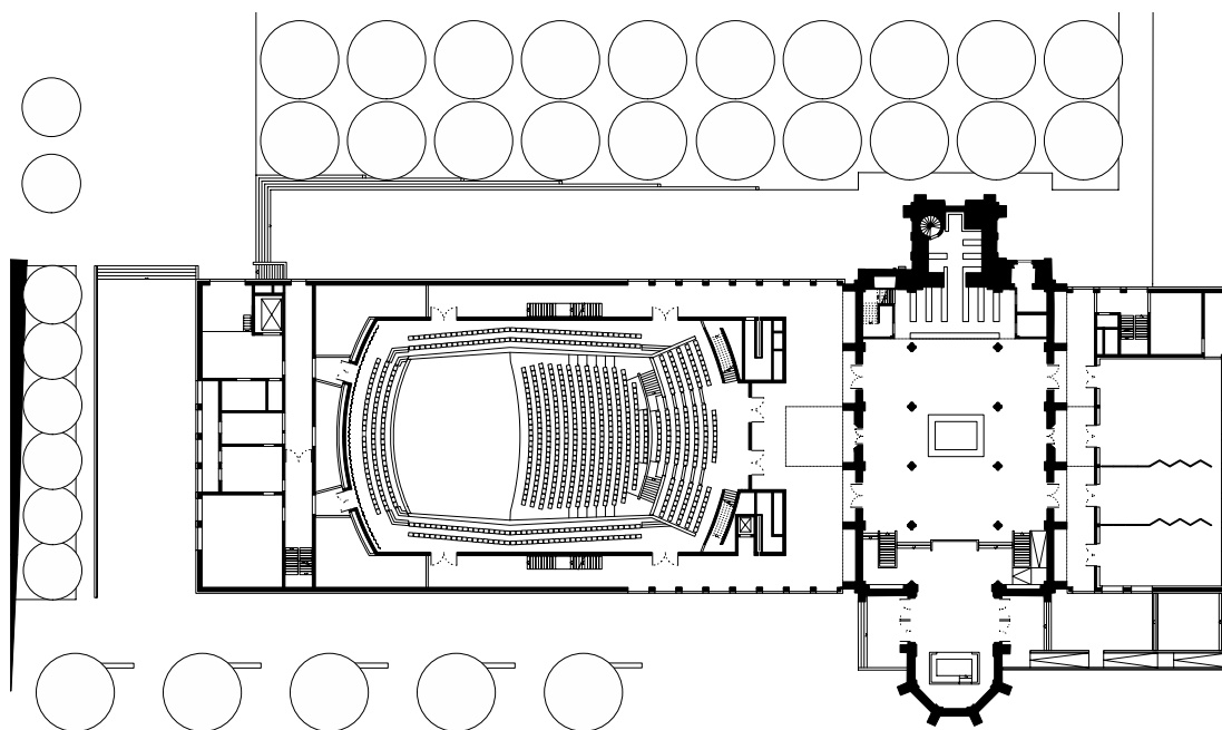
Grundriss Erdgeschoss
