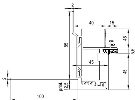
Dimenzioniranje okvirja vrat Zeroline
