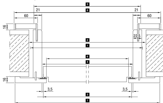
Vodoravni prerezi
