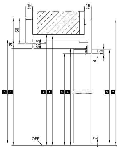
Navpični prerez
