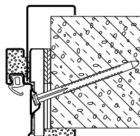
Za diagonalno pritrditev z dopolnilnim vratnim okvirjem Vario B53 kot 2-delni objemni vratni okvir (plinasti beton)
