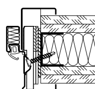
Za diagonalno pritrditev (plinasti beton)
