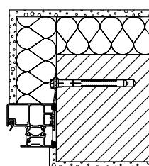
Fiksni vrtni okvir Montaža s sidri
