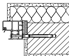
Fiksni vrtni okvir Vgradnja v zidano steno Montaža na špaletu
