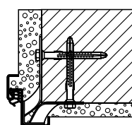
Vgradnja s sidri z moznikom
