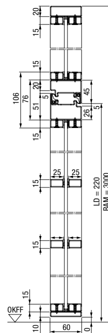
Navpični prerez 2-krilnih jeklenih loft vrat z obsvetlobami in nadsvetlobo
