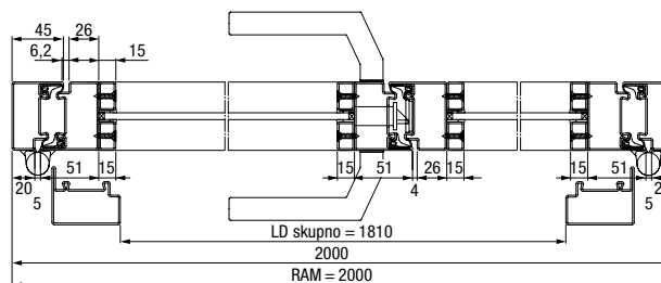
Vodoravni prerez 2-krilnih jeklenih loft vrat
