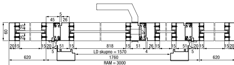
Horizontalni prerez 2-krilnih jeklenih loft vrat z obsvetlobami in nadsvetlobo
