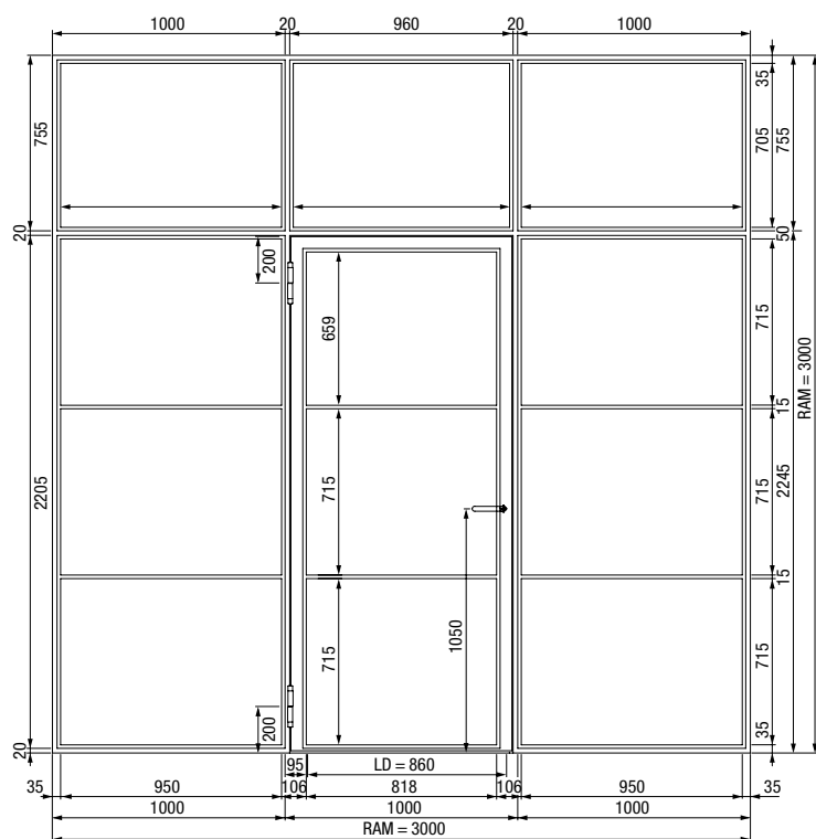
1-krilna jeklena loft vrata z obsvetlobami in nadsvetlobo
