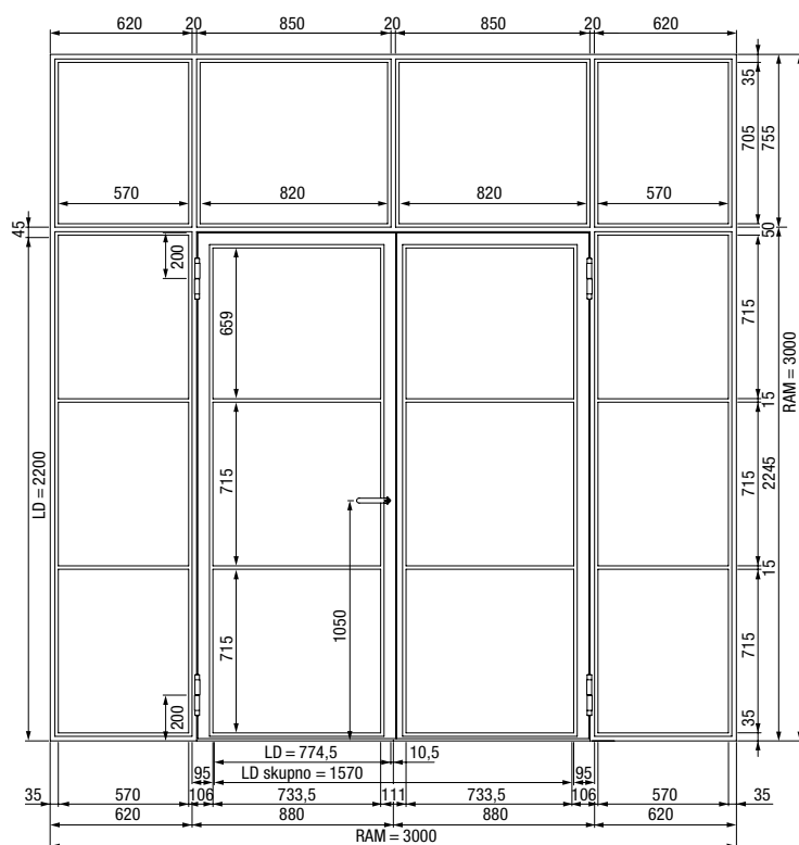
2-krilna jeklena loft vrata z obsvetlobami in nadsvetlobo
