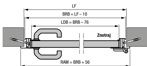
Stranska vrata z aluminijastim kotnim vratnim okvirjem s profilom tipa 1 ali 2 Pritrditev na notranji strani
