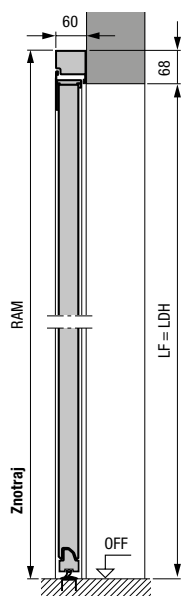
Stranska vrata z aluminijastim fiksnim vratnim okvirjem s profilom tipa 2 Vgradnja za odprtino
