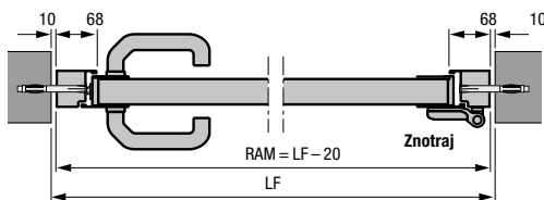
Stranska vrata z aluminijastim fiksnim vratnim okvirjem s profilom tipa 2 Vgradnja v odprtino
