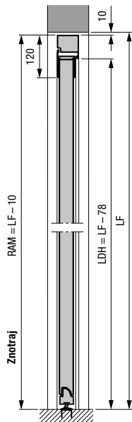
Stranska vrata z aluminijastim fiksnim vratnim okvirjem s profilom tipa 2 Vgradnja v odprtino
