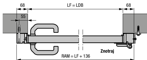
Stranska vrata z aluminijastim fiksnim vratnim okvirjem s profilom tipa 1 Vgradnja za odprtino
