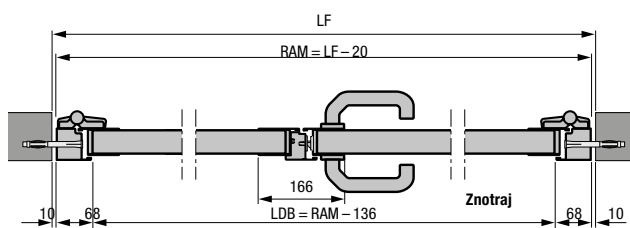
2-krilna stranska vrata z aluminijastim fiksnim vratnim okvirjem s profilom tipa 2 Vgradnja v odprtino
