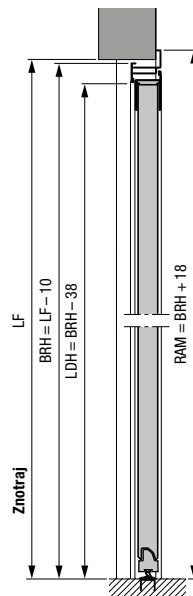
Stranska vrata z aluminijastim kotnim vratnim okvirjem s profilom tipa 2 Zunanji prislon
